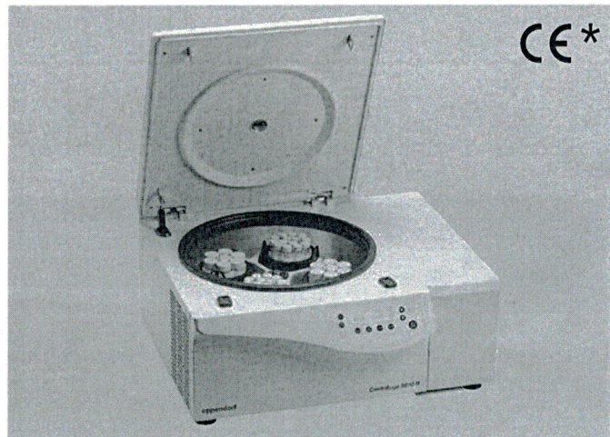
Centrifuge 5810 R con rotore S-4-104 (4 x 750 mL)
